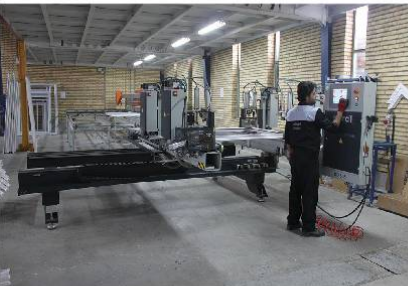
کنترل دمای محیط و صحت اطلاعات ورودی به دستگاه رباتیک چهار سر جوش پولیش
